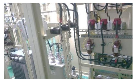
受電設備の2次側配線
