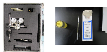
<圧縮空気中不純物測定セット>
